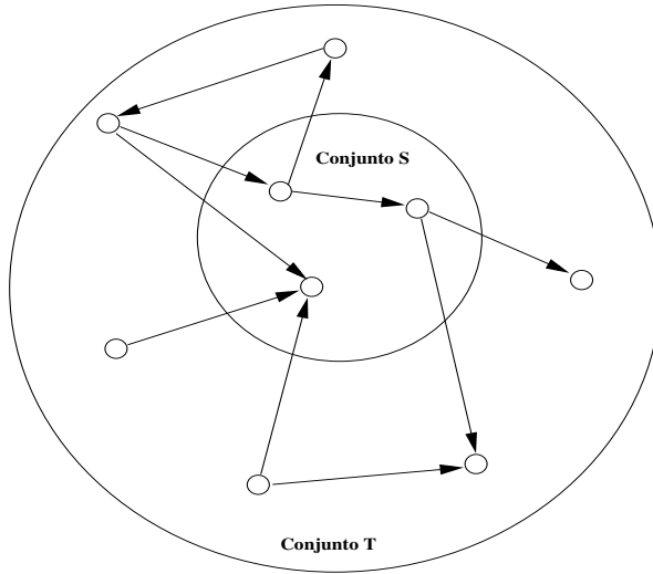
Figura 2. Conjuntos S e T utilizados pelo algoritmo HITS (adaptado a partir de [16])
