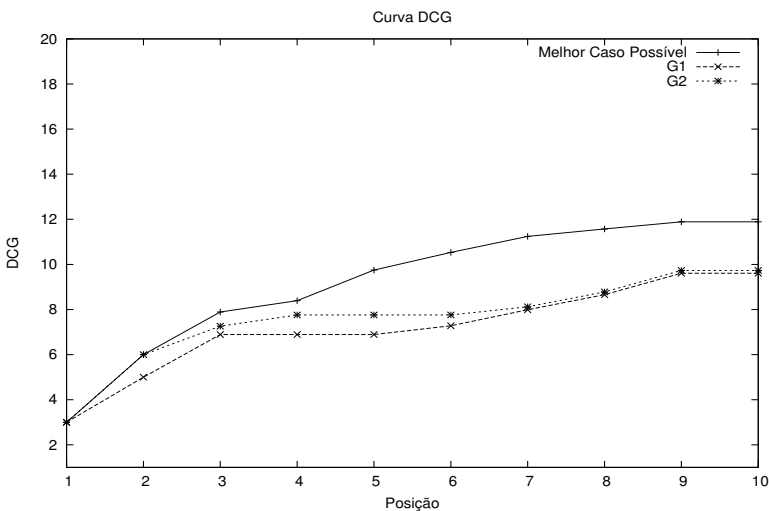
Figura 6. Exemplo de curva DCG
