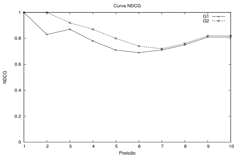
Figura 7. Exemplo de curva NDCG
